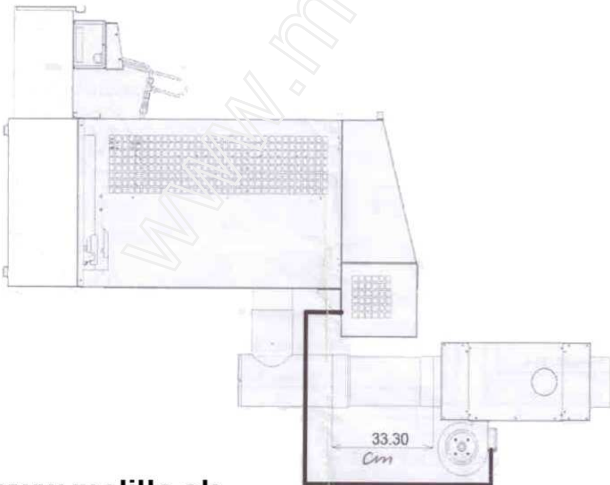
Pohľad na prepojenie Ekonomizéra
