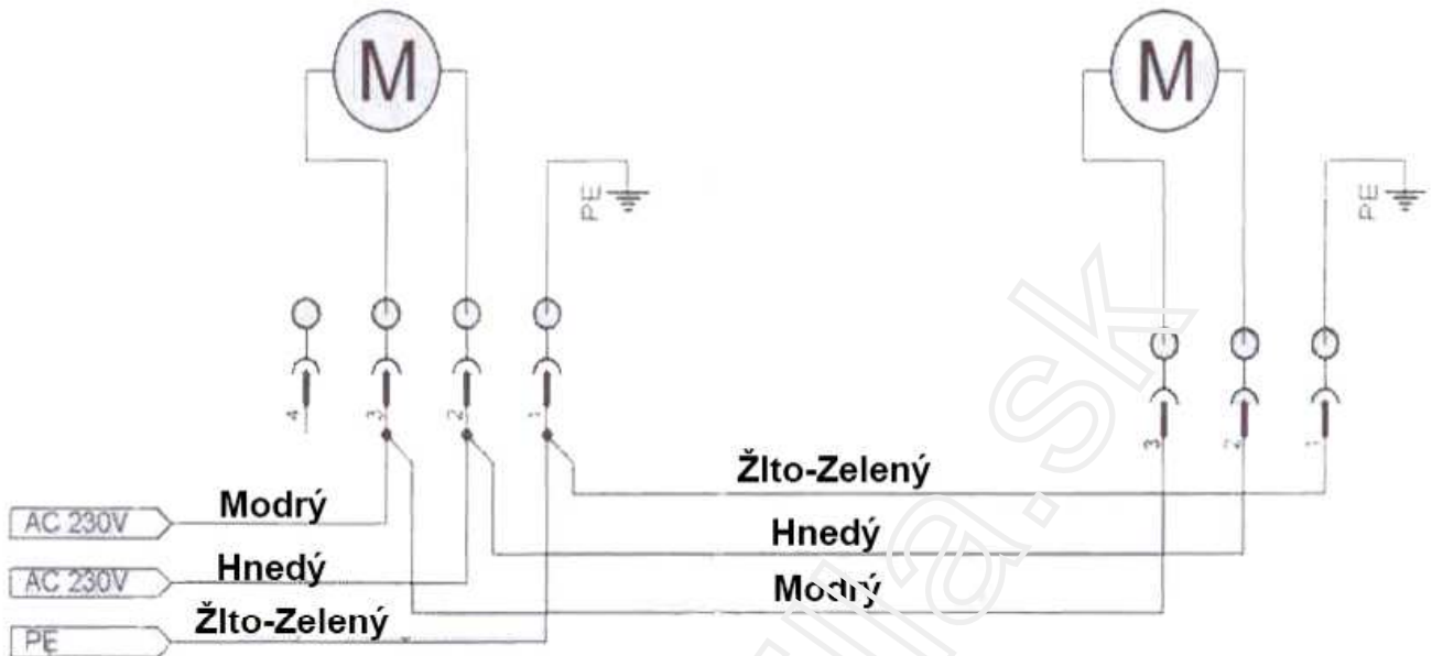
Ventilátor Ohrievača
